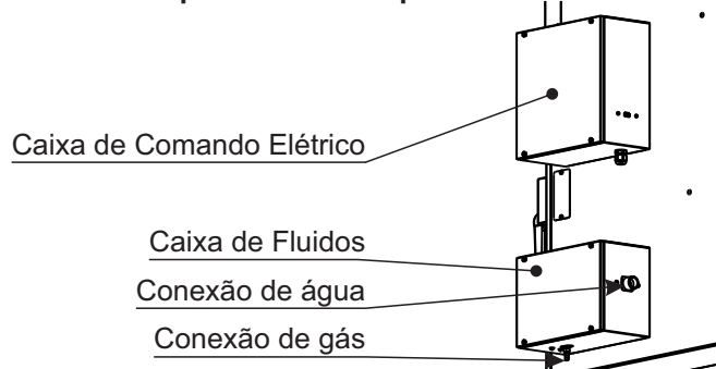
Figura 2: As caixas de comando elétrico e de fluidos são separadas para evitar acidentes.
